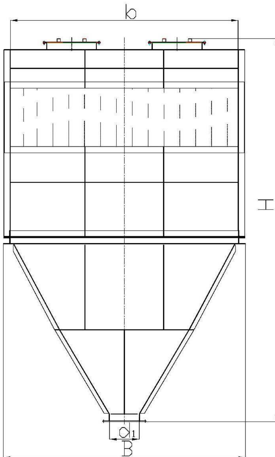
ТЕХНИЧЕСКИЕ ХАРАКТЕРИСТИКИ БАТАРЕЙНЫХ ЦИКЛОНОВ ЦБ
